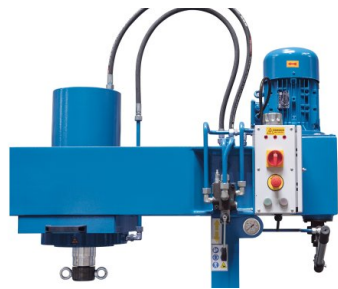
Cilindrul hidraulic este reglabil lateral pentru setarea simplă
